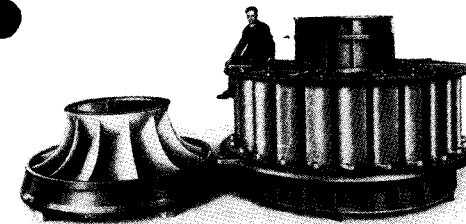
Lauf- und Leitrad einer Francis-Schachtelturbine mit stehender Welle
